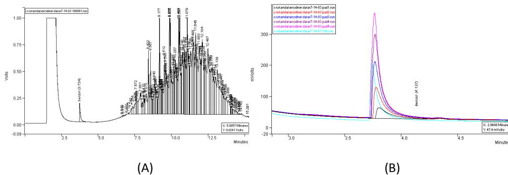
Figura 1: Cromatogramas obtidos a partir da injeção de 1 \mu L dos padrões e da amostra de medicamento conforme descrito anteriormente: (A) completo e (B) ampliado na região da banda do álcool benzílico.
